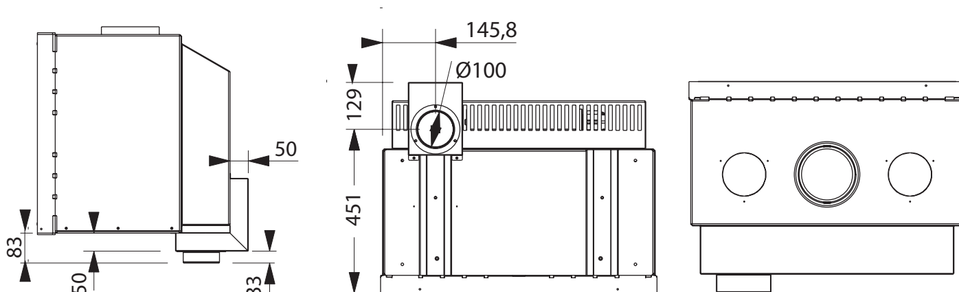
Inux 75 ventilato con presa aria inferiore /Ventilated with inferior air intake
